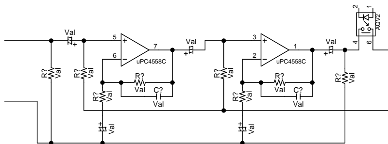
書きかけ回路図・・・PDFの表示サンプル用
